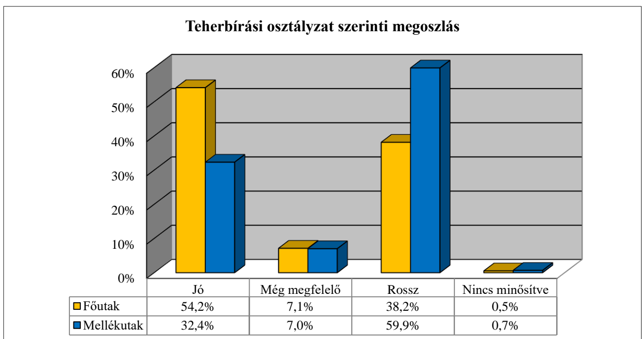
5. diagram: Teherbírési osztályzat szerinti megoszlás
