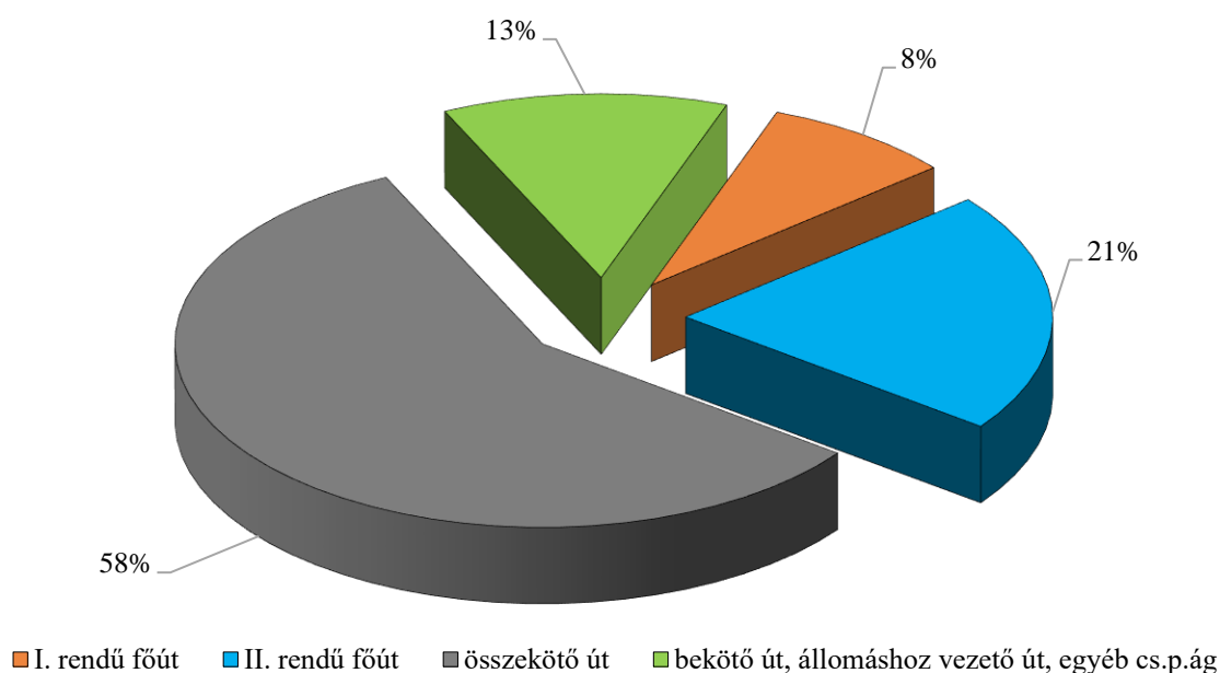
1. diagram: A vármegyei országos közúthálózat útkategóriánkénti bontásban
