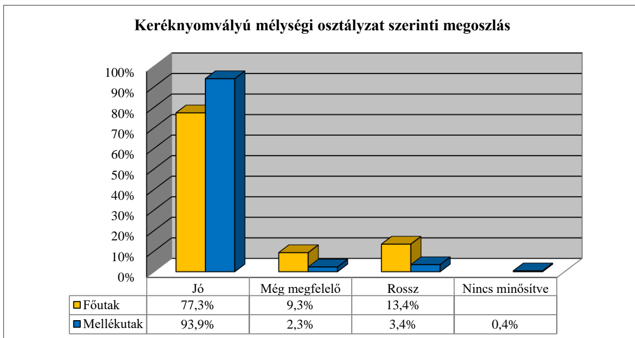
9. diagram: Keréknyomvályú mélységi osztályzat szerinti megoszlás
